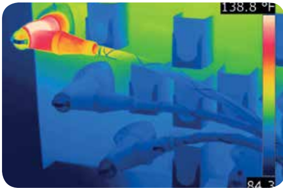
Exx AŞIRI ISINMIŞ KONEKTÖR
